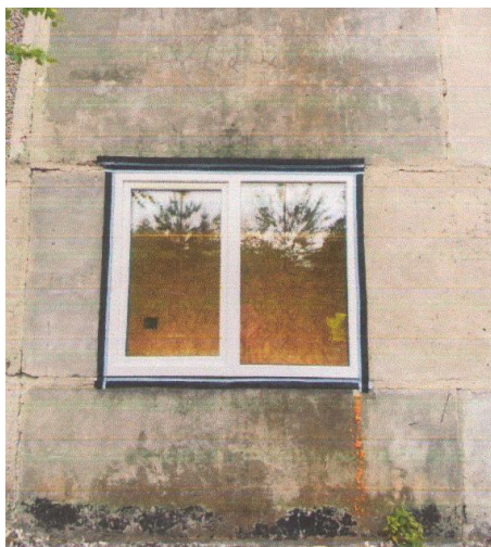
Рис. 4. Віконна конструкція зразка №S2-02_2023 до (ліворуч) та після (праворуч) випробування [8]
