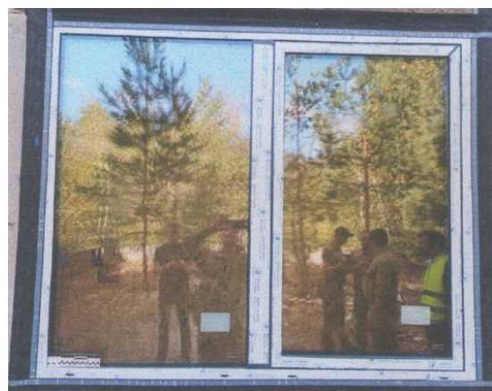
Рис. 6. Віконна конструкція зразка №S3-02_2023 до (ліворуч) та після (праворуч) випробування [6]
