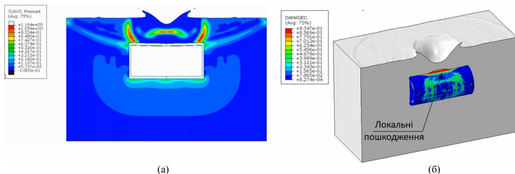
Рис. 8. Вплив вибухової ударної хвилі на модифіковану конструкцію укриття:
