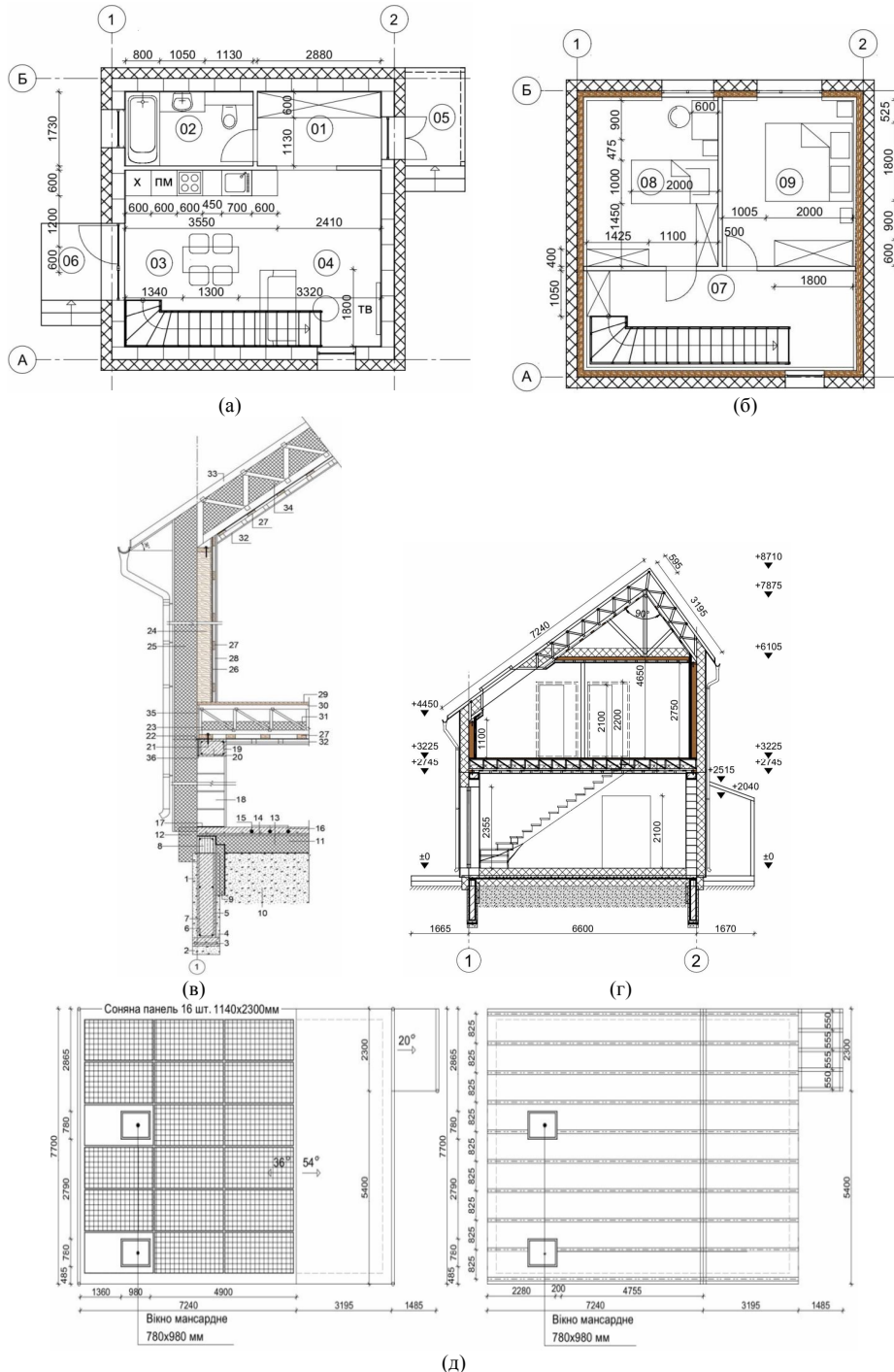
Рис. 1. Архітектурно-планувальне рішення будинку Start TM “Business House” за стандартом NZEB: (а) план першого поверху; (б) план другого поверху; (в) розріз по стіні; (г) розріз будинку; (д) план кроквяних ферм та покрівлі з фотопанелями сонячної електростанції
