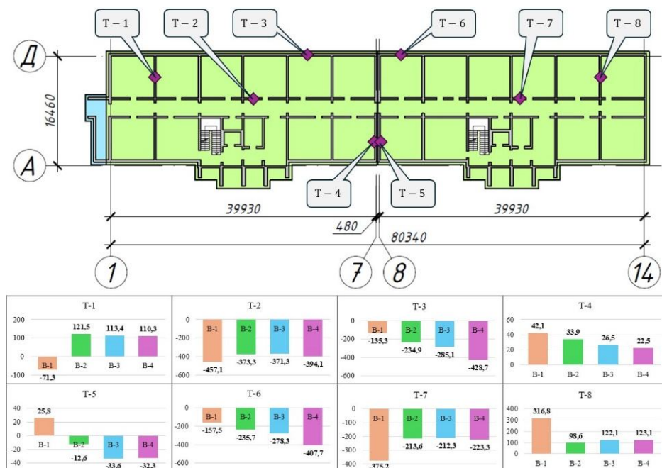
Рис. 11. Горизонтальні напруження у фундаментних стінах, кПа
