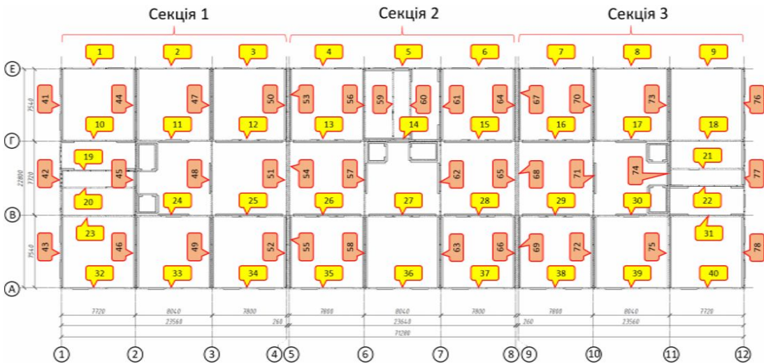
Рис. 4. Нумерація стінових панелей для аналізу результатів розрахунків
