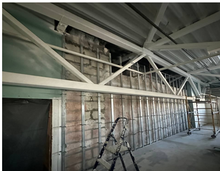
Рис. 6. Відновлена частина ферми та покриття
