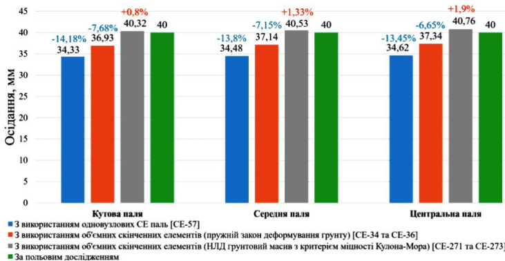
Рис.9. Порівняння осідань характерних паль на останній стадії навантаження (1800кН)
