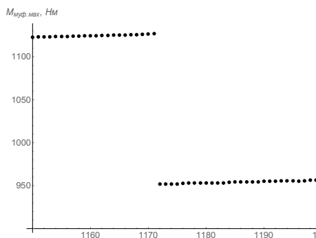
Рис. 9. Графік зміни максимального моменту M_{\text{муф, макс}} у муфті в залежності від коефіцієнта дисипації
