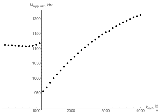
Рис. 7. Графік зміни максимального моменту M_{муф \text{ max}} у муфті в залежності від коефіцієнта дисипації
